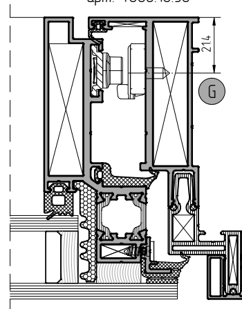
Установка ответной планки арт. 4060.10.50
