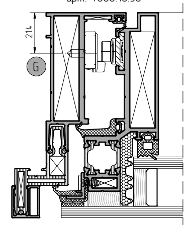
Установка ответной планки арт. 4060.10.50
