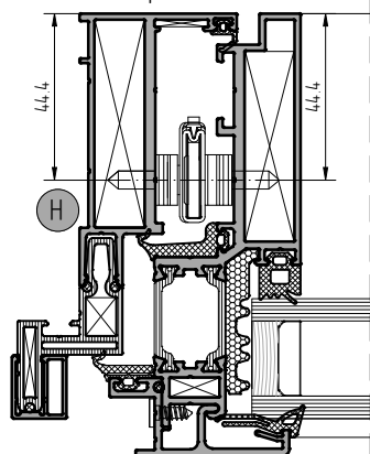
Установка ограничителя открывания арт. 4060.10.50
