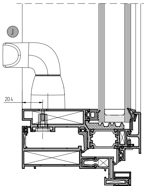
Установка поводковой ручки арт. 1107.10R и арт. 1107.10L
