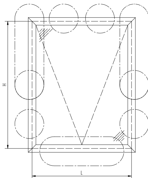
Установка поводковой ручки арт. 1107.10R и арт. 1107.10L
