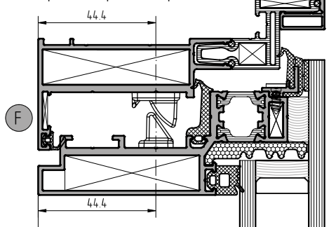
Установка скрытого верхнего прижима арт. 4060.45
