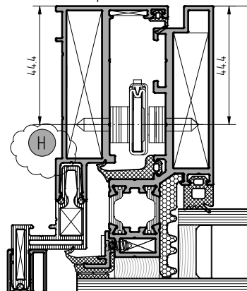
Установка ограничителя открывания арт. 4065.30
