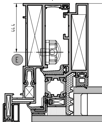
Установка ответной планки арт. 4060.10.50
