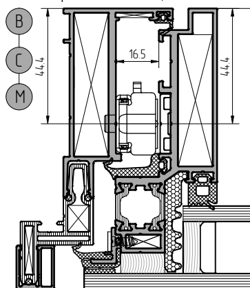
Установка механизма регулировки по высоте арт. 4060.04
