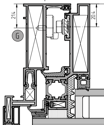
Установка ограничителя открывания арт. 4065.30
