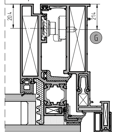
Установка ограничителя открывания арт. 4065.30
