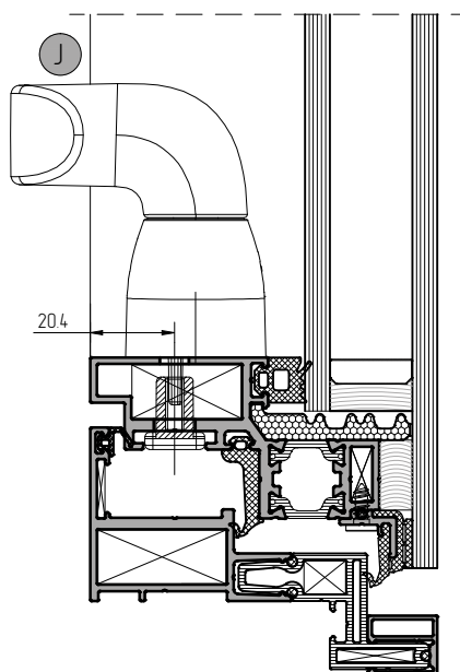
Установка поводковой ручки арт.1107.10R и арт.1107.10L
