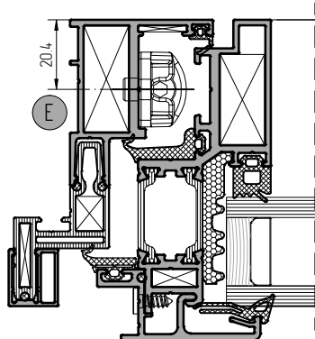
Установка ответной планки арт. 4060.10.50
