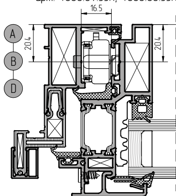
Установка механизма регулировки по высоте арт.4060.04
