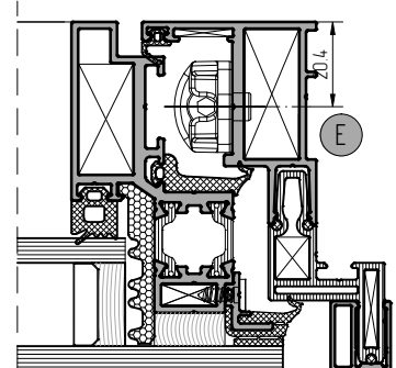
Установка механизма регулировки по высоте арт.4060.04
