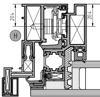
Установка ограничителя открывания арт. 4065.00
