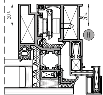
Установка ограничителя открывания арт. 4065.00
