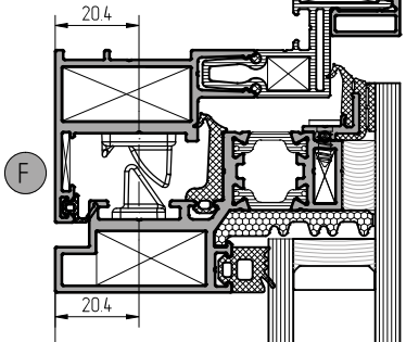
Установка скрытого верхнего прижима арт. 4060.45
