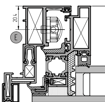
Установка механизма регулировки по высоте арт.4060.04
