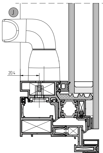
Установка поводковой ручки арт.1107.10R и арт.1107.10L
