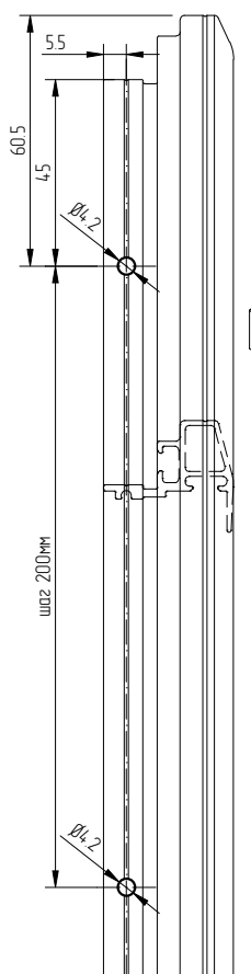
Профиль опорный под стеклопакет АУРС.F50.1823
