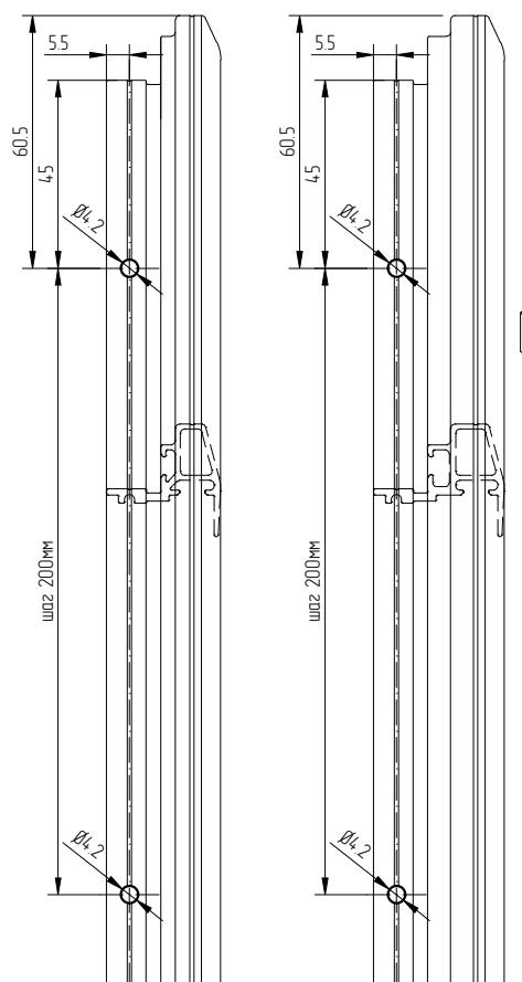
Профиль опорный под стеклопакет АУРС.F50.1822
