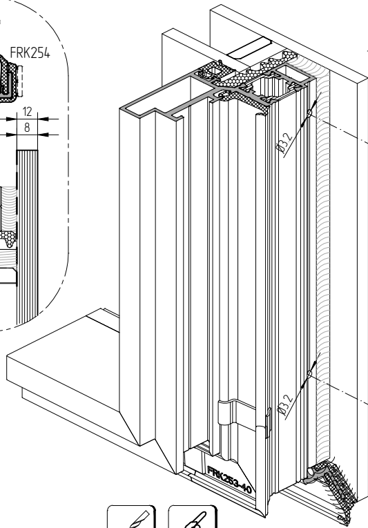
Профиль опорный под стеклопакет АУРС.F50.1815
