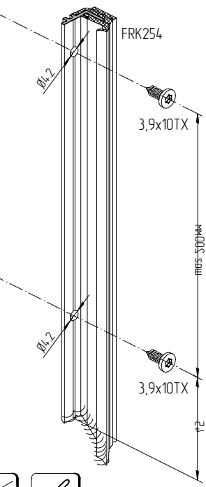
Профиль опорный под стеклопакет АУРС.F50.1815
