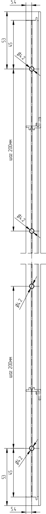
Профиль опорный под стеклопакет АУРС.F50.1815
