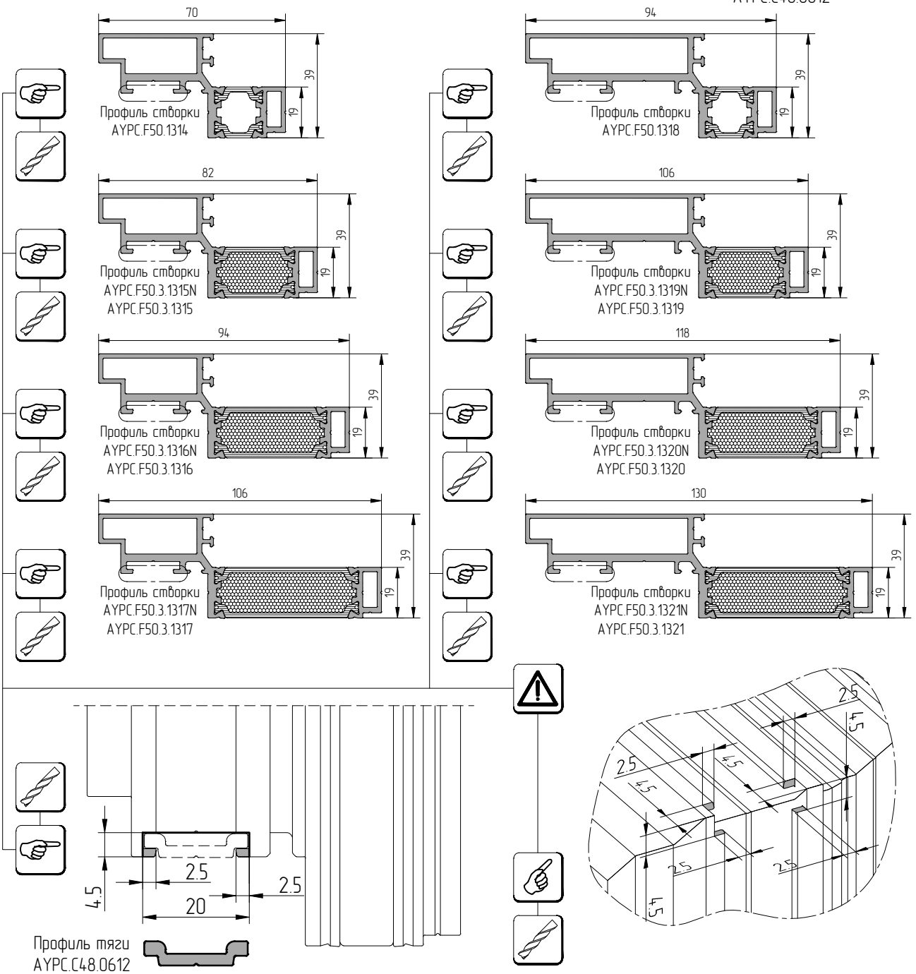
Профиль тяги АУРС.С48.0612
