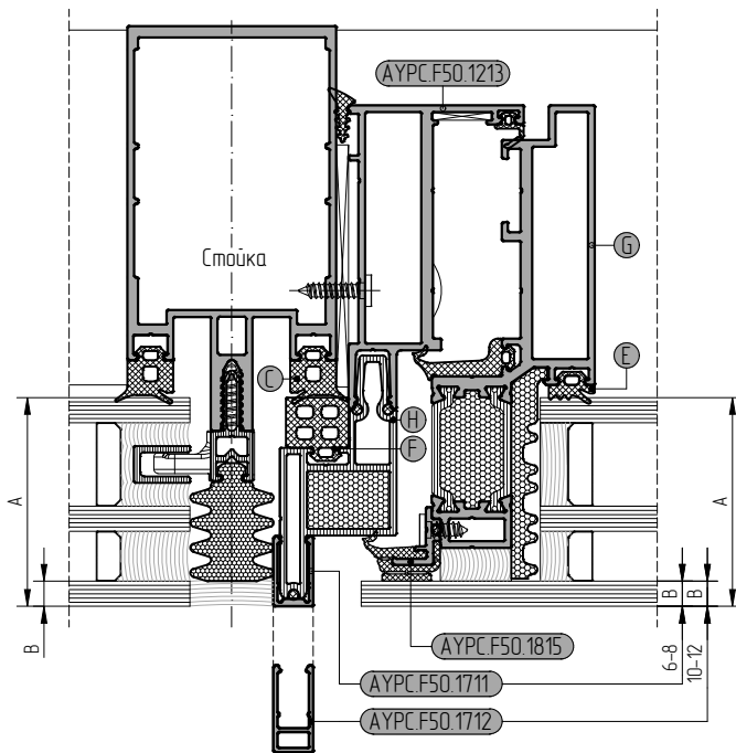
Сечение через стойку
