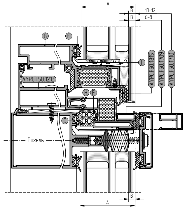
Сечение через ригель
