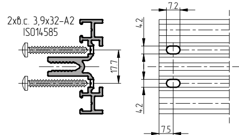
Обработка ригеля АУРС.F50.0231
