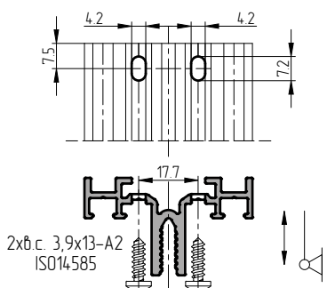
Обработка ригеля АУРС.F50.0231 в зависимости от способа установки
