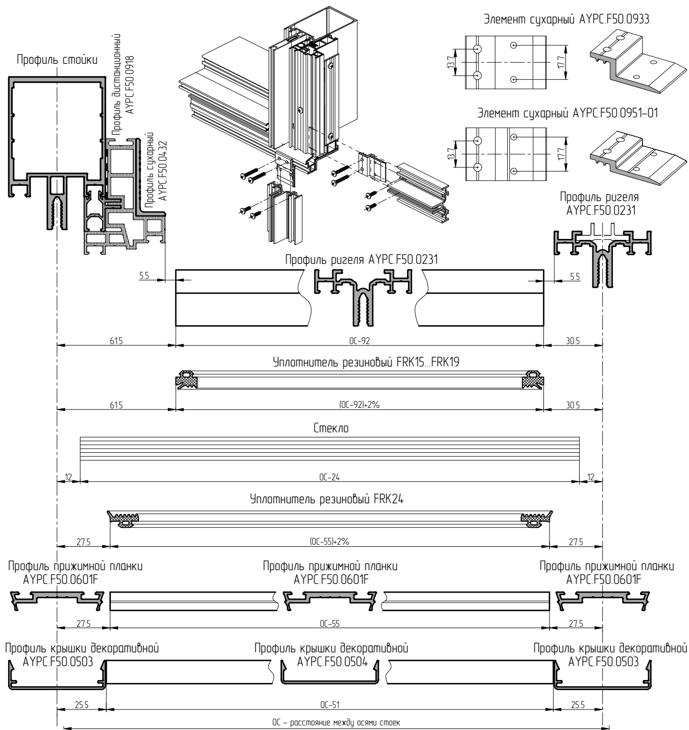
Обработка ригеля АУРС.F50.0231 в зависимости от способа установки
