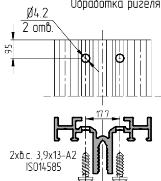
Обработка ригеля АУРС.F50.0231 в зависимости от способа установки
