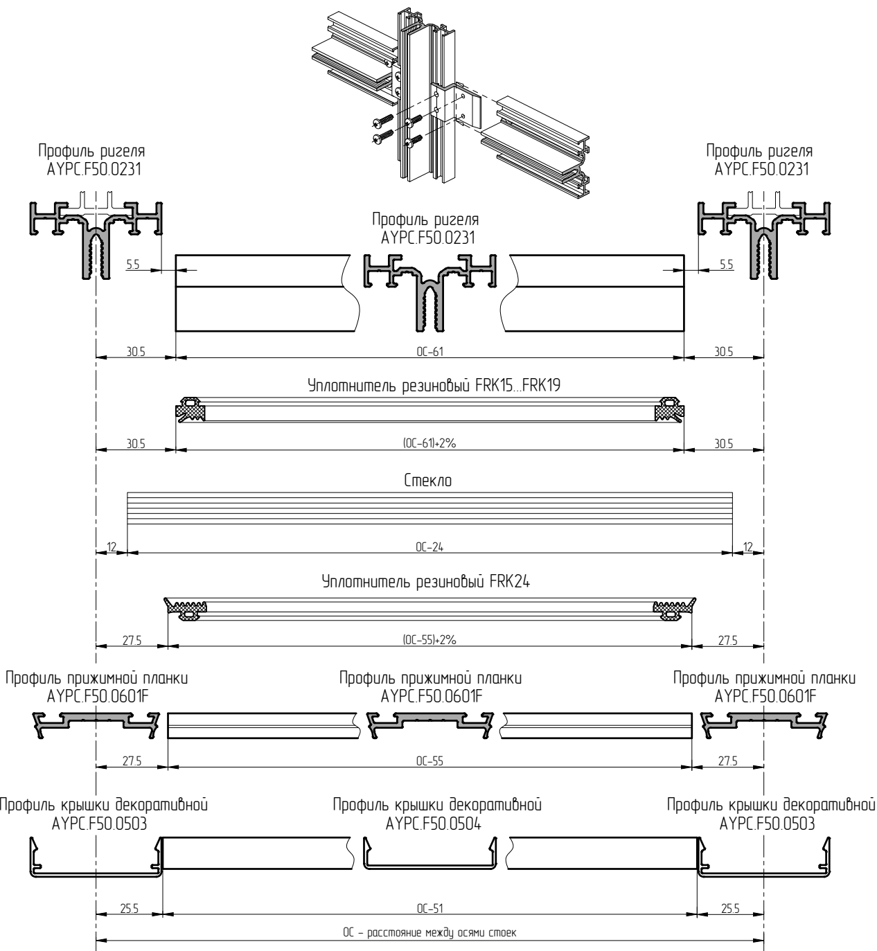
Обработка ригеля АУРС.F50.0231
