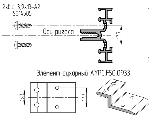
Обработка ригеля АУРС.F50.0231
