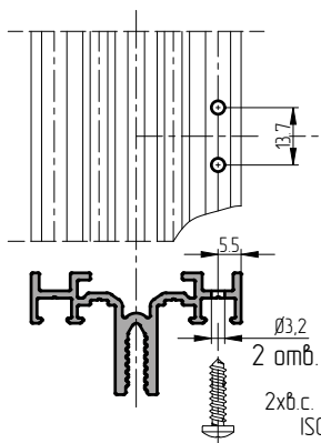
Обработка ригеля АУРС.F50.0231
