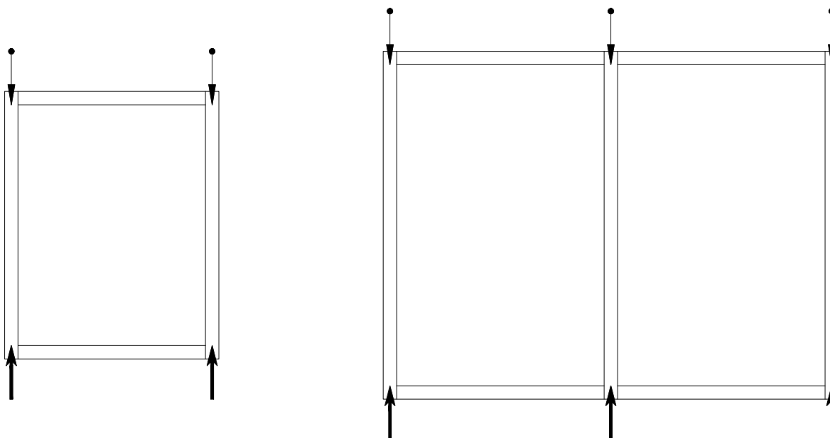
Схема расположения опор системы ALT F50HC на каркасе "теплой" области витража
