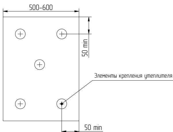
Схема крепления утеплителя на углу здания
