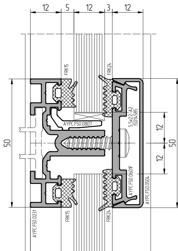
Вариант 1 Ригель соединяется со стойкой
