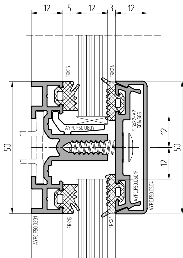
Вариант 2 В качестве стойки используется ригель
