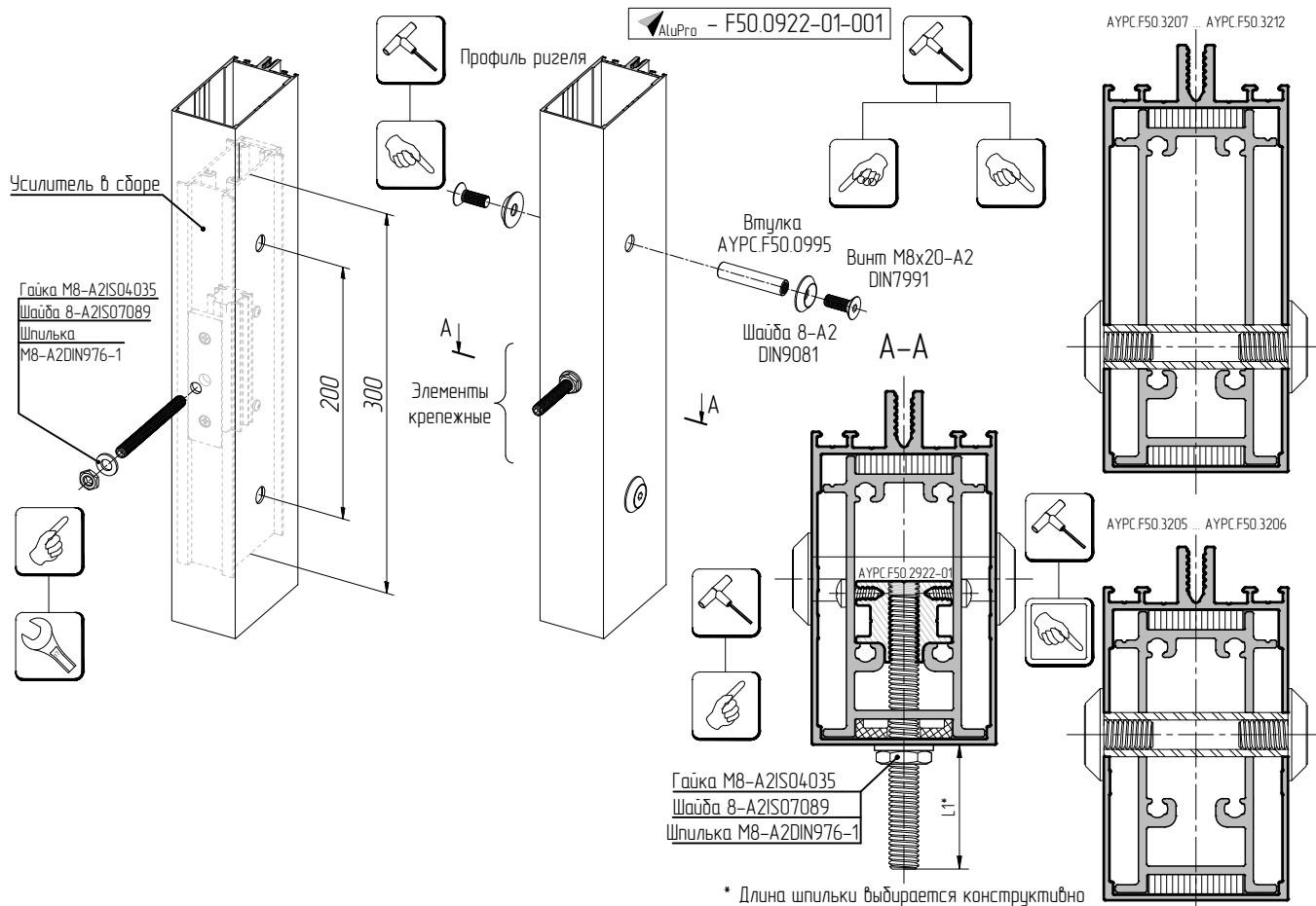
Обработка профиля стойки / ригеля
