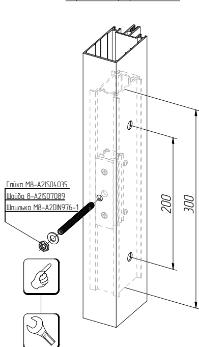
Обработка профиля стойки
