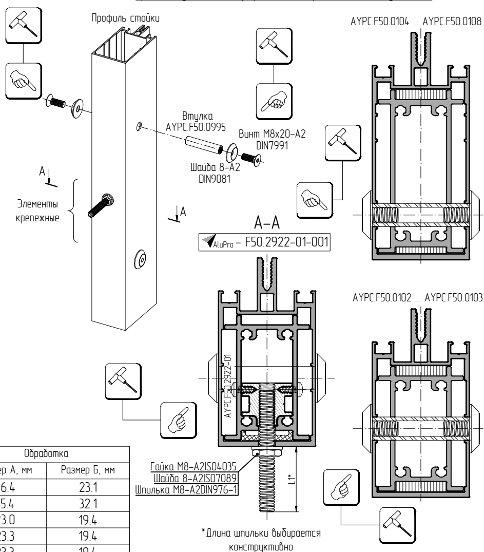
Крепление усилителя в профиле стойки при его локальной установке
