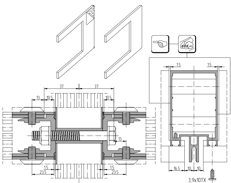
Вариант В \blacktriangledown AluPro – ВНС-05/C+ С установкой мягких резиновых заглушек ригеля
