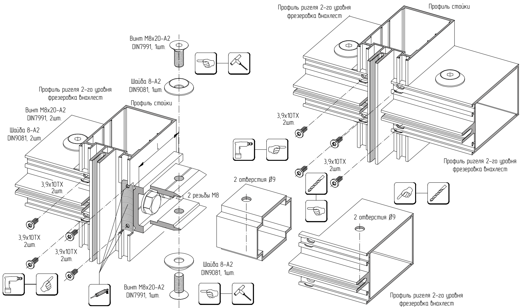
Вариант А \blacktriangledown AluPro – ВНС-05/A+ Без установки заглушек ригеля
