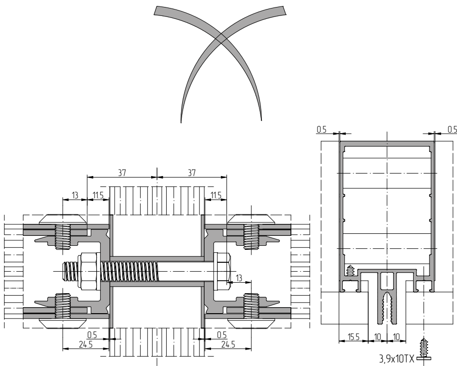
Вариант А \blacktriangledown AluPro – ВНС-05/A+ Без установки заглушек ригеля
