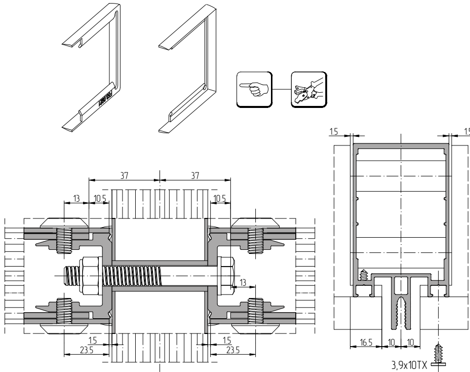
Вариант Б \blacktriangledown AluPro – ВНС-05/B+ С установкой пластиковых заглушек ригеля
