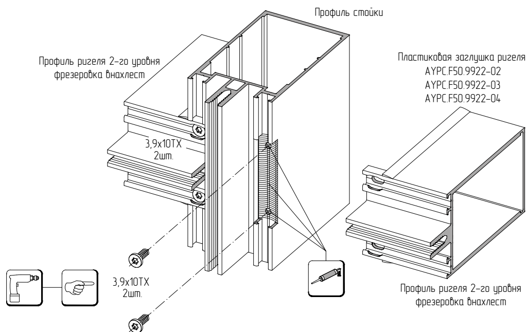
Вариант А | ▲AluPro – ВНС-01/А
