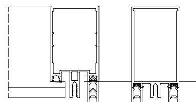
Ригель внахлест
