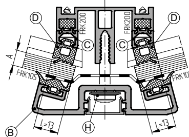
Стойка с двусторонним углом разворота
