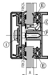
Ригель внахлест
