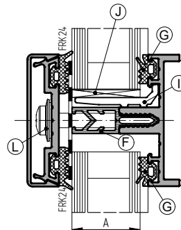
Ригель внахлест
