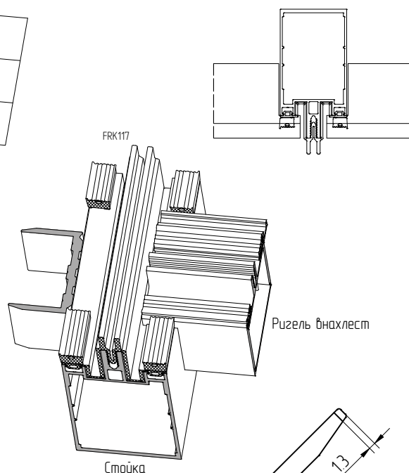
Стойка
