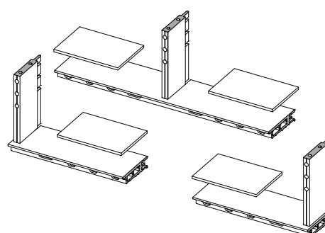
Тип опорных подкладок 3
