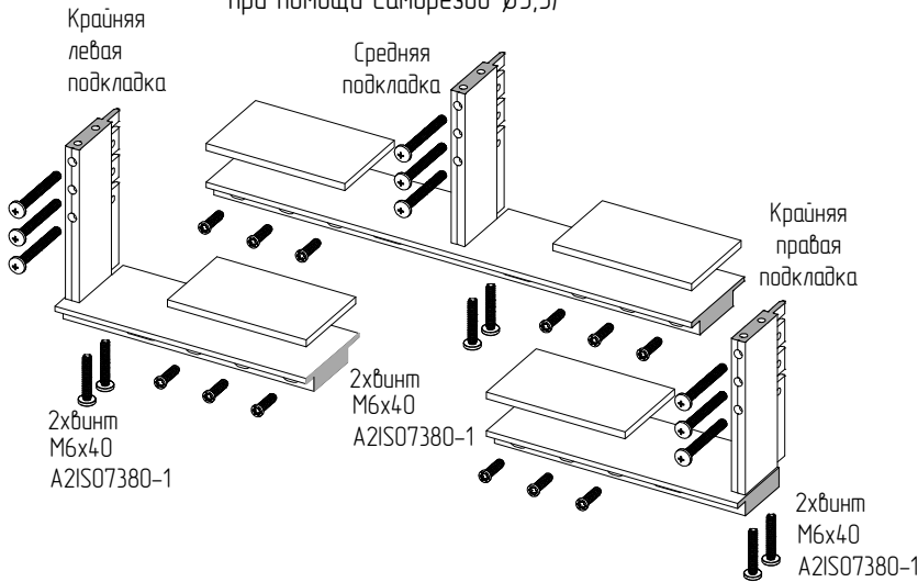
Крепление крестообразной опорной подкладки ТИП 3
