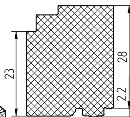
Подрезка для профиля АУРС.F50.0740
