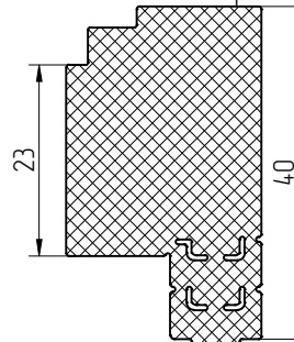
Подрезка для профилей АУРС.F50.1936, АУРС.F50.1937
