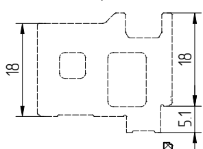
Подрезка для профилей АУРС.F50.1936, АУРС.F50.1937
