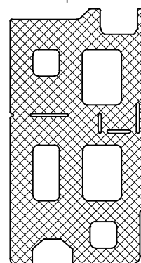
Для профилей АУРС.F50.1938, АУРС.F50.1939 деталь не подрезается
