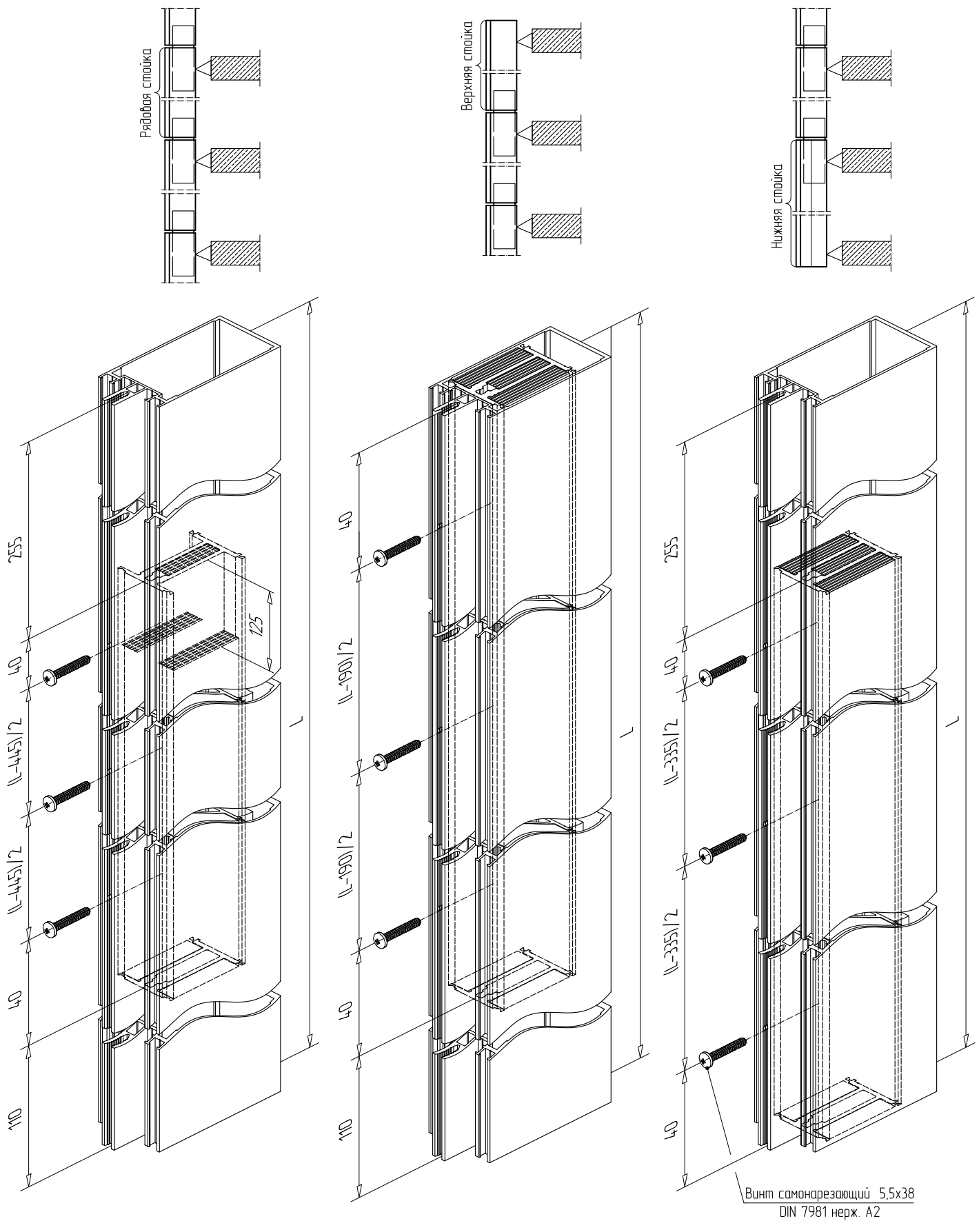
Схема установки усиливающего профиля в стойку EI 45.
