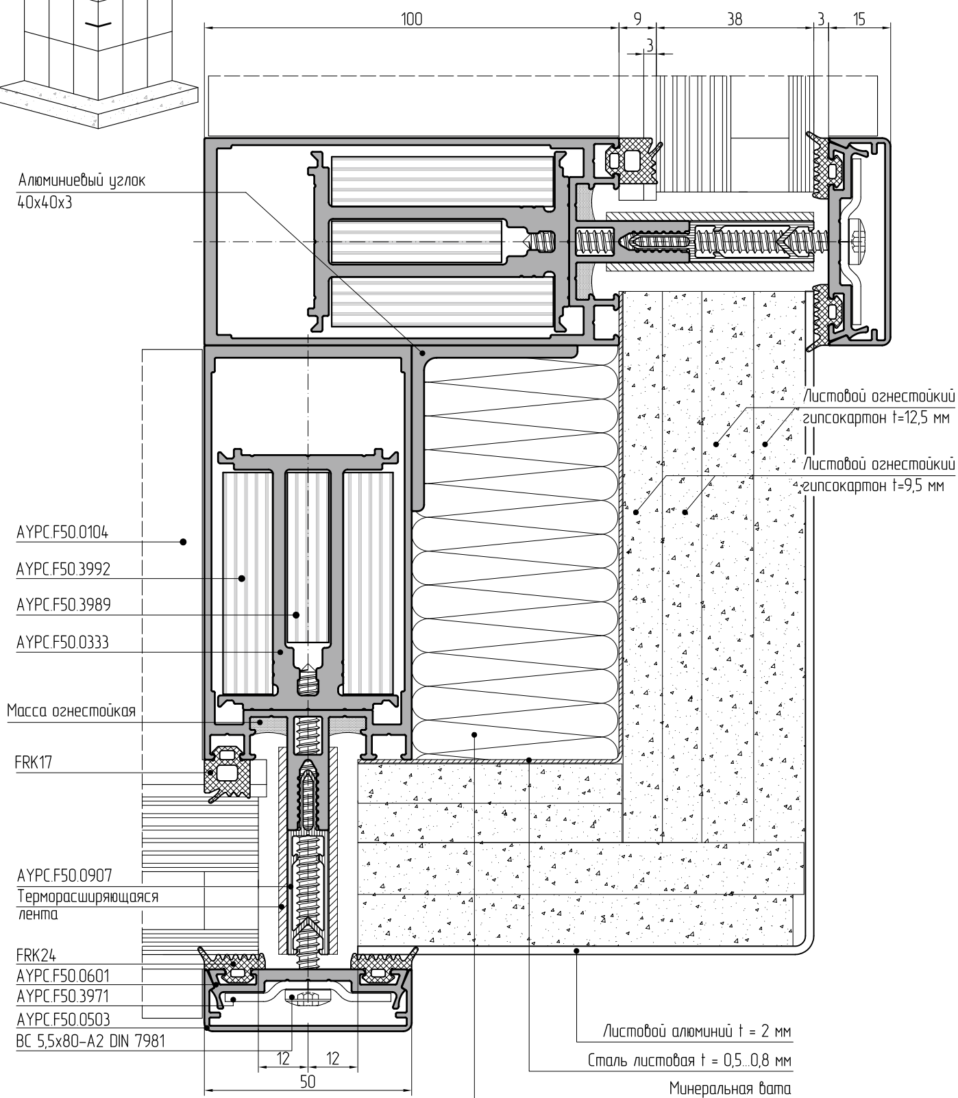
Сечения EI 45
