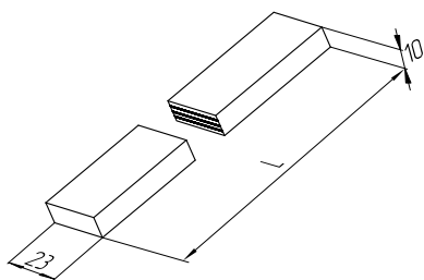
Вставка огнестойкая
