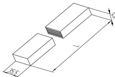
Вставка огнестойкая
