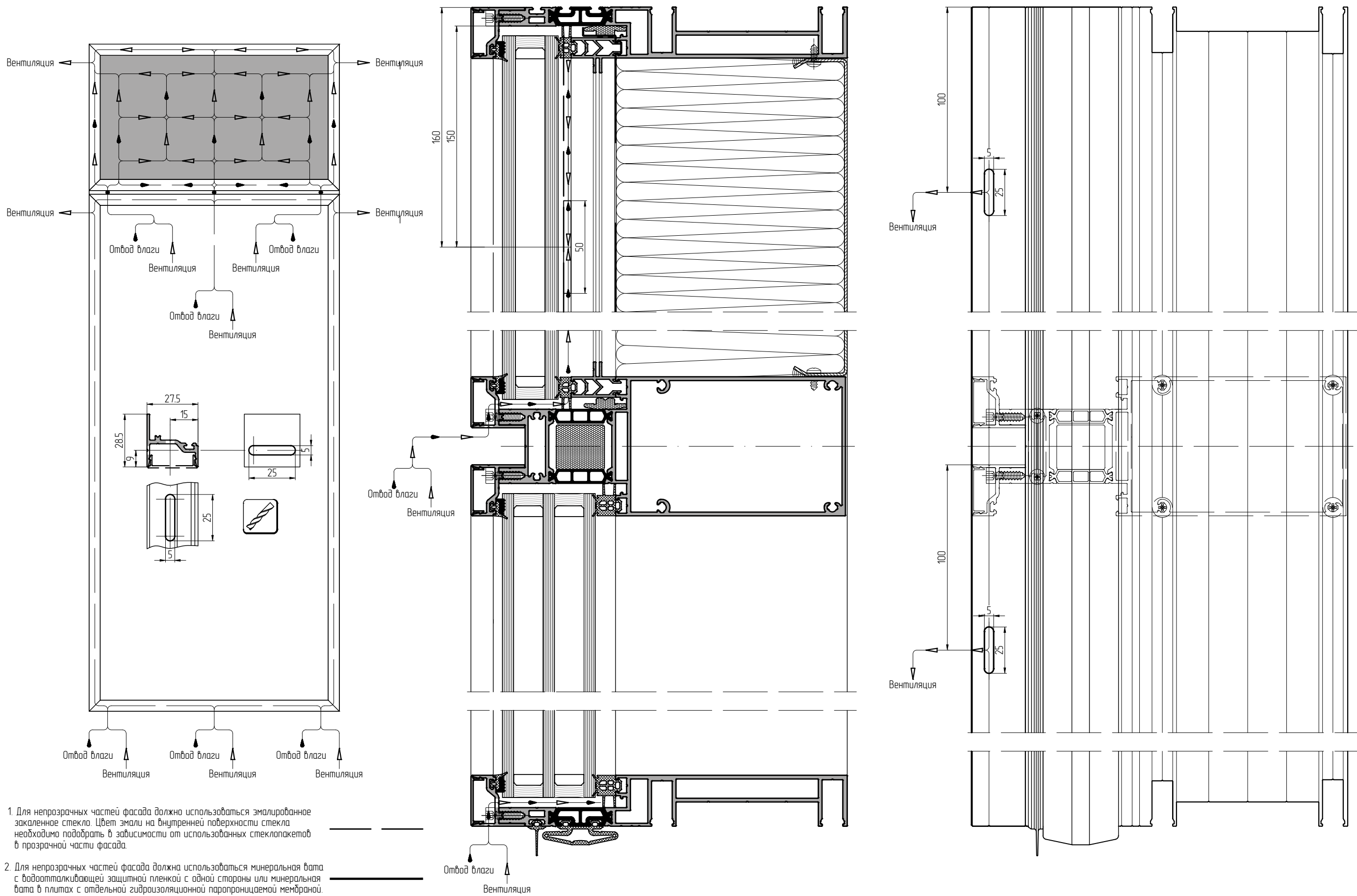
Схема вентиляции и отвода влаги из области фальца стеклопакета для прямой прозрачной и непрозрачной части конструкции фасада
