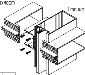
Ригель внахлест
