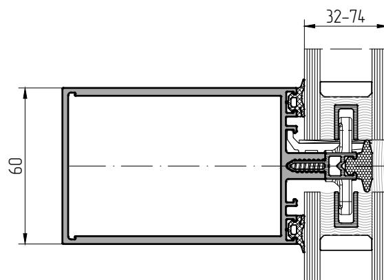
Сечение конструкции по ригелю
