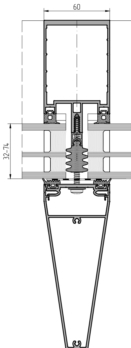
Сечение конструкции по стойке
