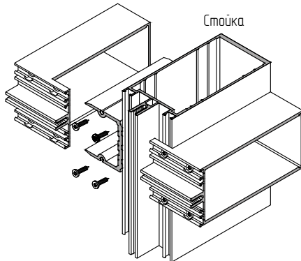
Ригель внахлест
