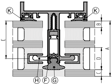
Ригель внахлест
