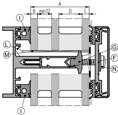
Ригель 2-го уровня фрезеровка внахлест
