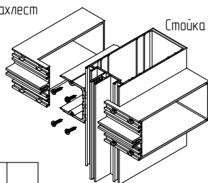
Ригель внахлест
