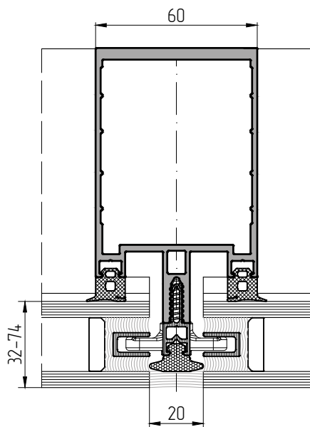
Сечение конструкции по стойке
