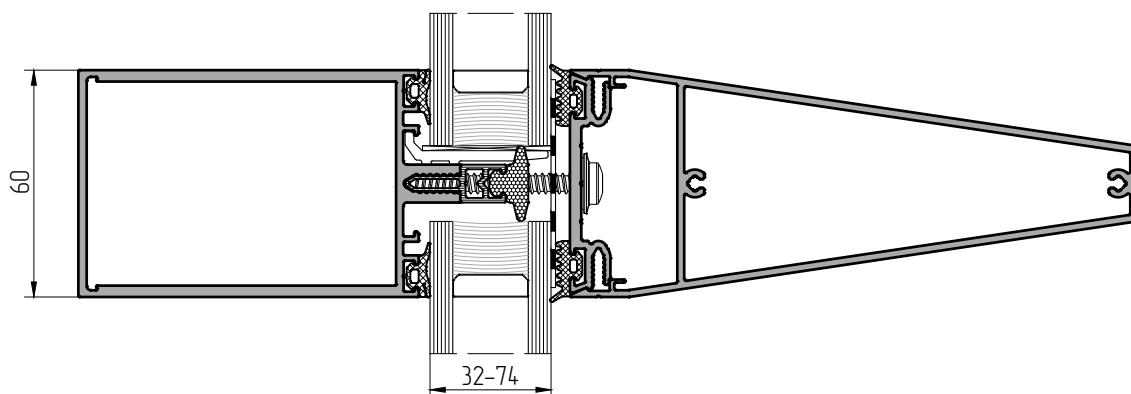
Сечение конструкции по ригелю
