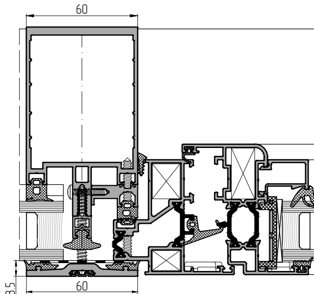
Однокамерный стеклопакет со встроенным оконным блоком
