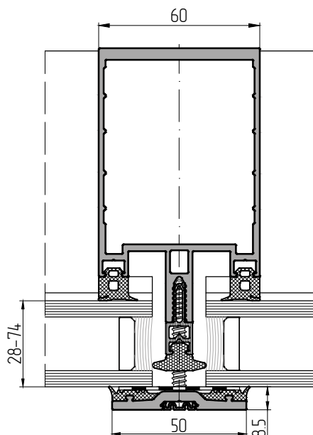
Однокамерный стеклопакет с декоративной крышкой из алюминиевого профиля
