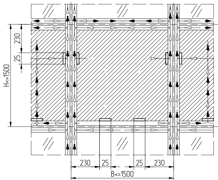
Обработка профилей АУРС.F50.2061 под установку угловых закладных АУРС.F50.5138
