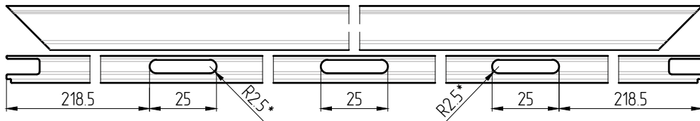
Обработка профилей АУРС.F50.2061 для вентиляции и отвода влаги
