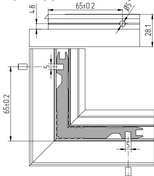
Обработка профилей АУРС.F50.1707 для вентиляции и отвода влаги
