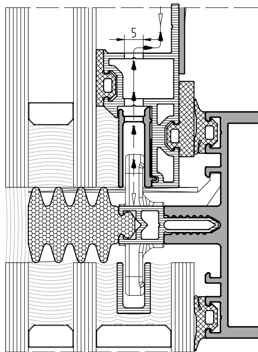
Схема расположения дренажных и вентиляционных отверстий
