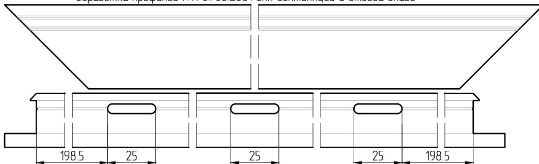
Обработка профилей АУРС.F50.2061 для вентиляции и отвода влаги
