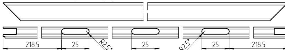
Обработка профилей АУРС.F50.1935 для вентиляции и отвода влаги
