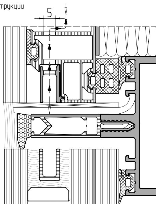
Обработка профилей АУРС.F50.2060 под установку угловых закладных АУРС.F50.5138
