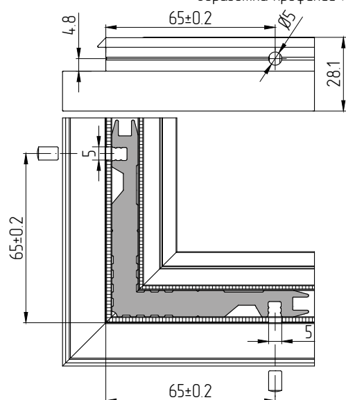
Обработка профилей АУРС.F50.1706 для вентиляции и отвода влаги
