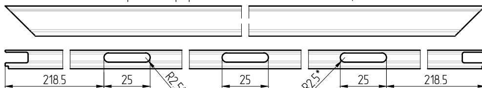
Обработка профилей АУРС.F50.2060 для вентиляции и отвода влаги
