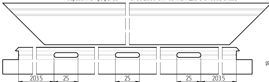
Обработка профилей АУРС.F50.2060 для вентиляции и отвода влаги
