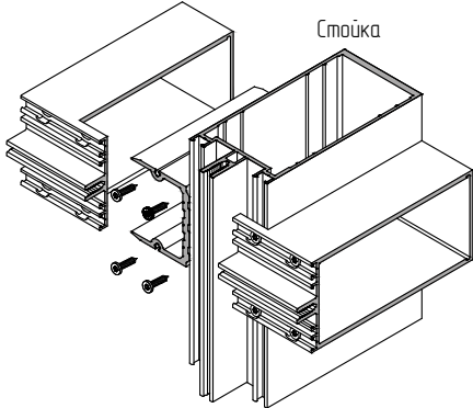
Ригель внахлест
