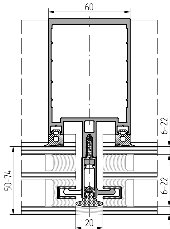
Двухкамерный стеклопакет с фиксацией за наружную камеру
