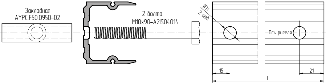
Закладная крепления ригеля, изгот. из профиля АУРС.F60.0401
