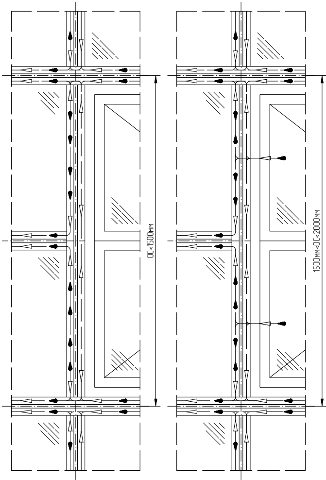
Схема вентиляции и отвода влаги из области фальца стеклопакета для прямой прозрачной части конструкции фасада
