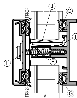
Ригель внахлест
