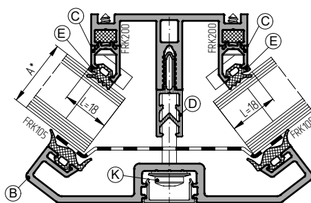
Стойка с двусторонним углом разворота
