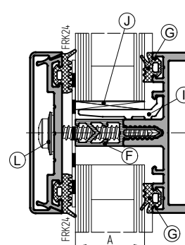
Ригель внахлест
