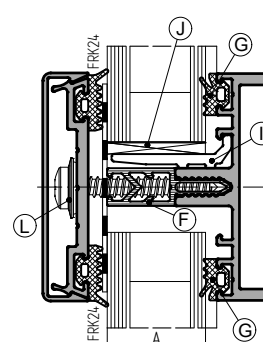
Ригель внахлест
