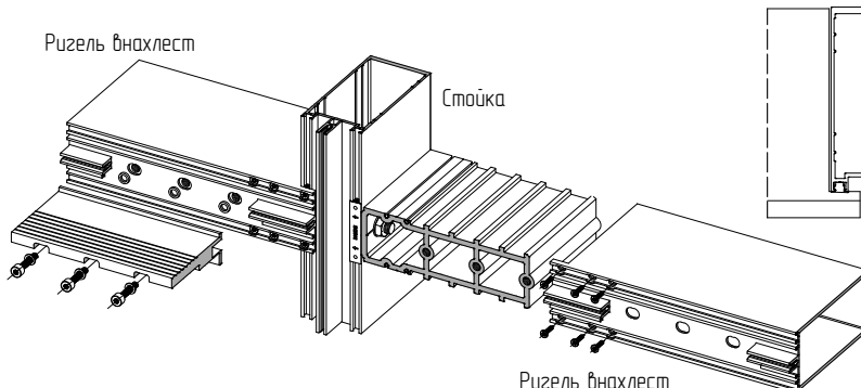
Ригель внахлест
