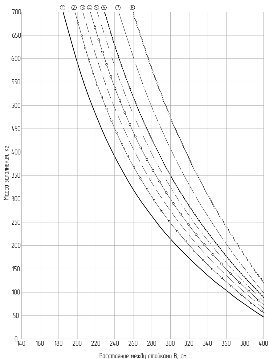
Типы опорных подкладок
